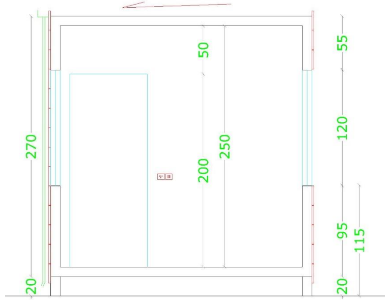
مقطع أ - أ
